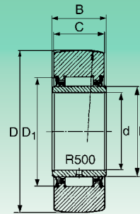
NA 22...2RS
