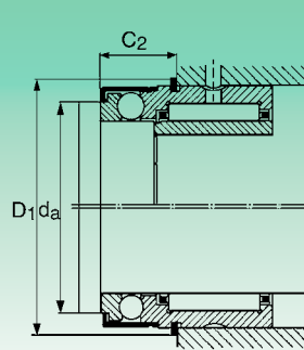
Dimensiones de montaje Mounting dimensions
